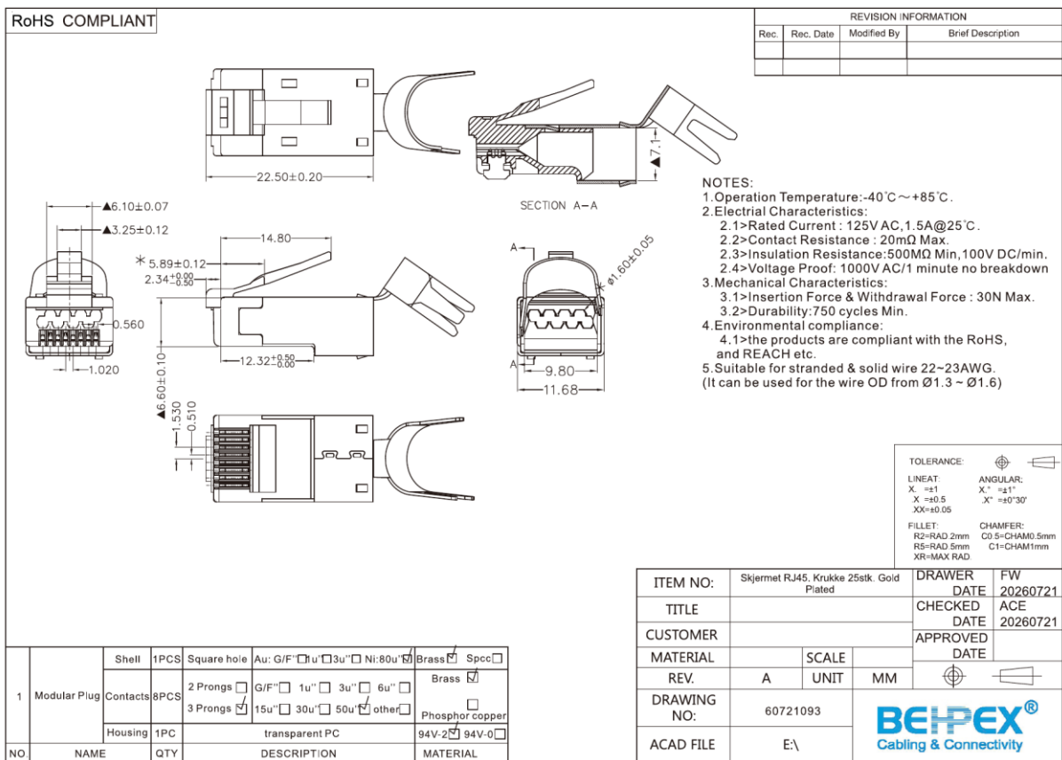
Figur 1: Plugg, samlet – mål i mm
