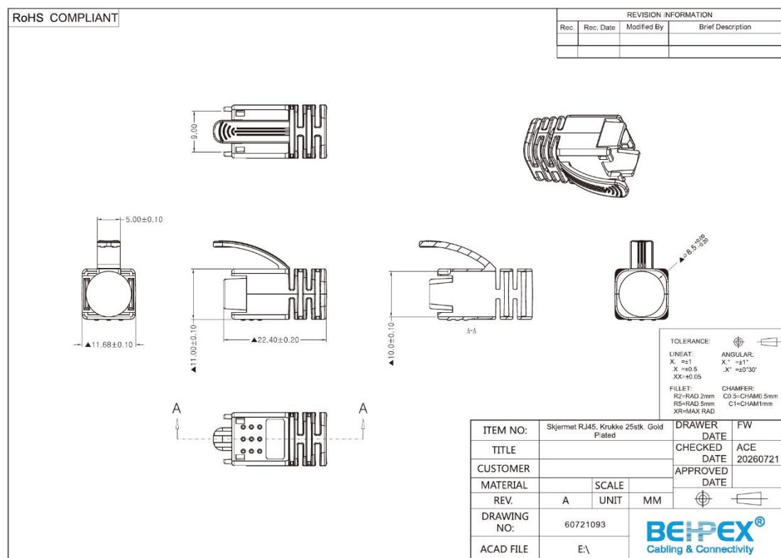
Figur 3: Streckkavlastning/kabelklemme – mål i mm
