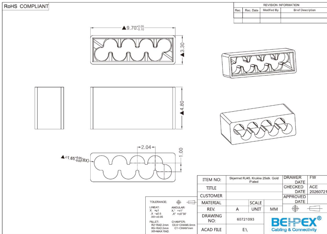
Figur 2: Lastbrikke (leder-organisator) – mål i mm
